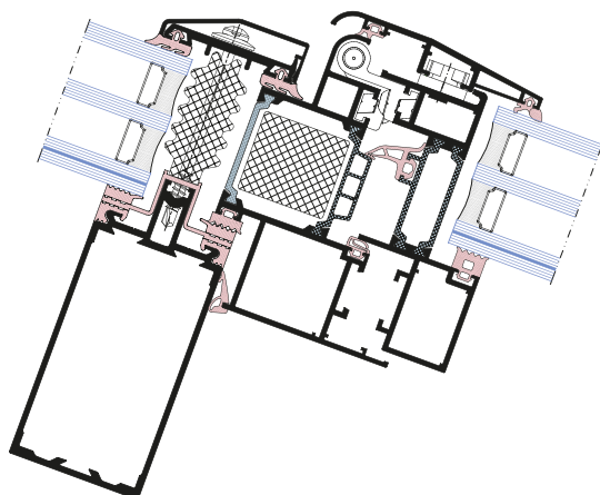
Okno dachowe AF 50R w fasadzie AF 50
