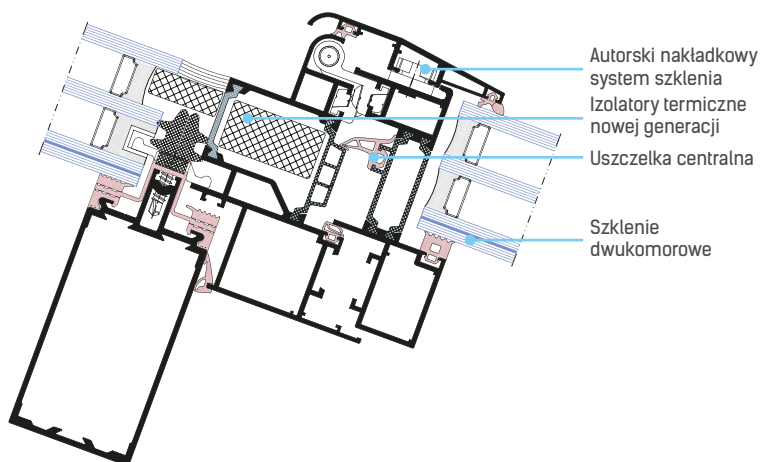
Okno dachowe AF 50R w fasadzie AF 50S
