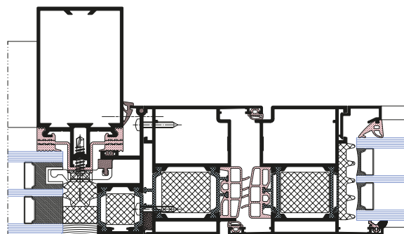
Połączenie fasady z drzwiami
