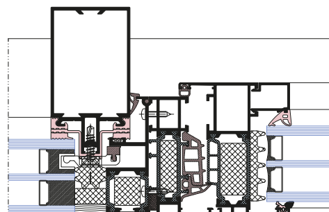
Połączenie fasady z oknem
