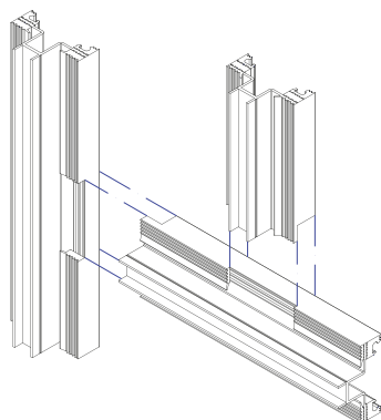
3 poziomy odwodnienia przy użyciu uszczelki płaszczej
