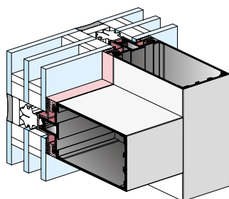
Licowanie profili i uszczelki od wewnętrznej strony fasady
